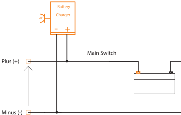
Abbildung 6. Anschluss eines Ladegerätes an die Batterie
